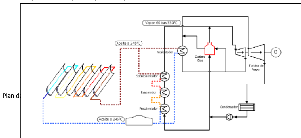
Figura 1.5 Esquema proceso productivo
