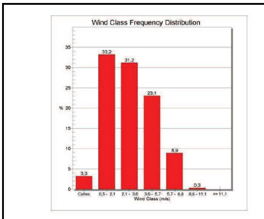
Figura 1.4.3.7.3. Frecuencia de velocidad del viento
