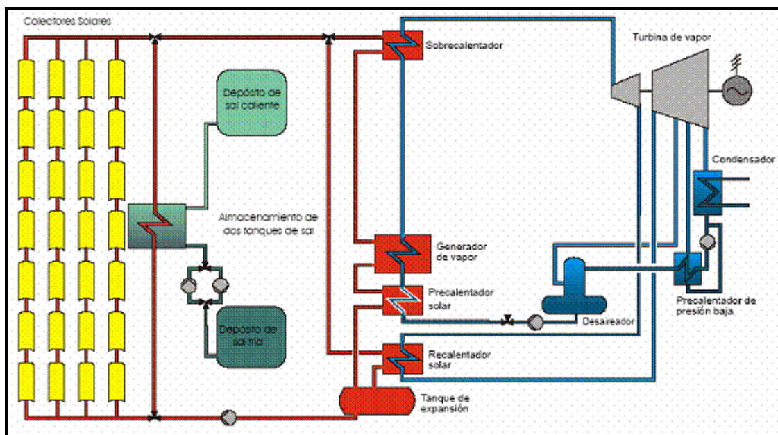
Figura 1.5.2. Esquema de funcionamiento de la Planta Termosolar
