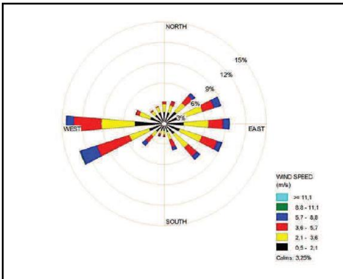
Figura 1.4.3.7.4: Rosa de los vientos
