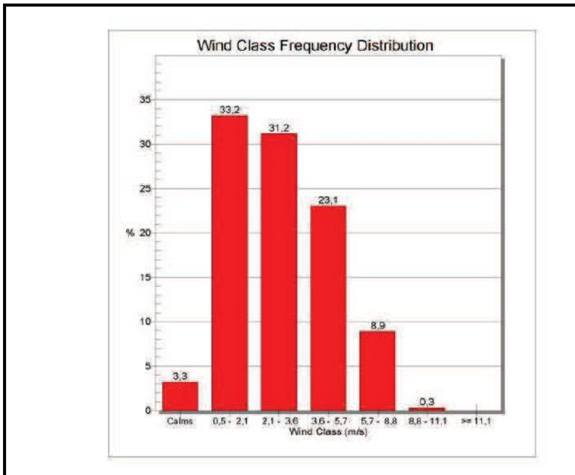
Figura 1.4.3.7.3. Frecuencia de velocidad del viento
